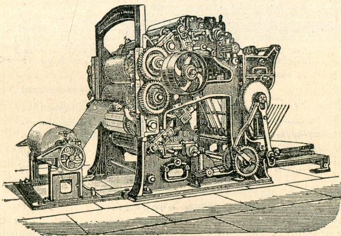
Ротаційна машина.
