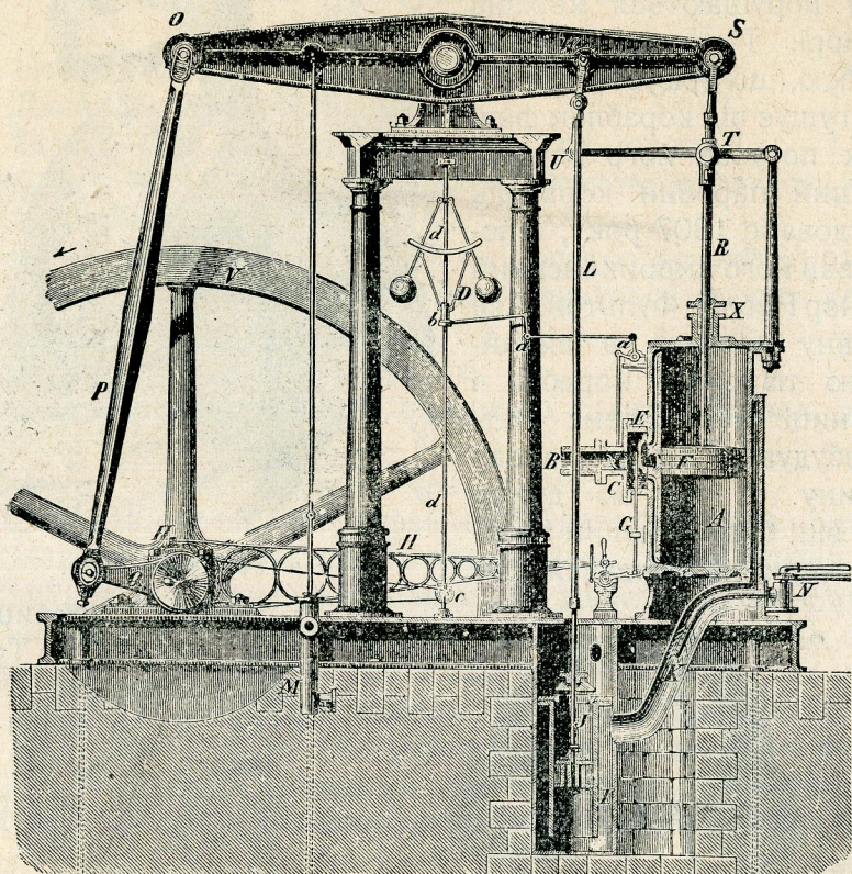
Вигляд парової машини сконструованої Джемсом Ватом:
