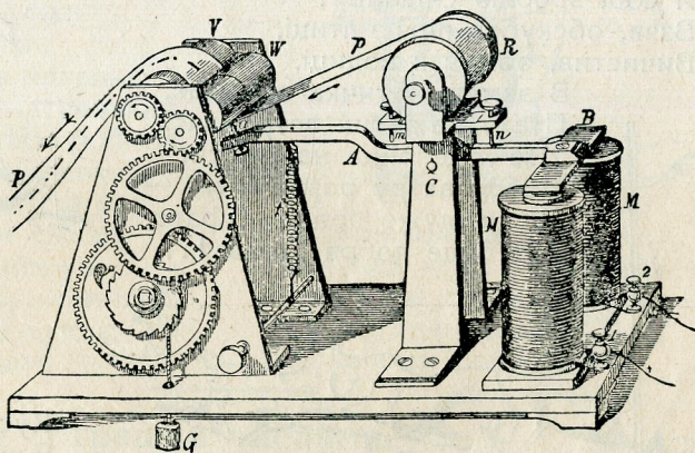
Апарат Морса
