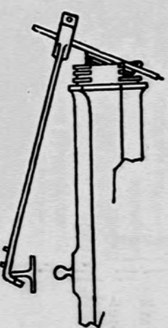
2. Ersatz des Griffstückes durch Lauf- und Visierkorrschlüssel.
