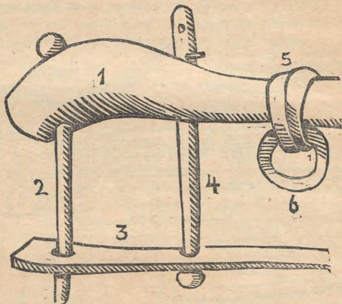
Рис. X. Ярмо: 1 = лутиці; 2 = завіски; 3 = підгорлиці; 4 = сніз (снози); 5 = привій; 6 — облук.
