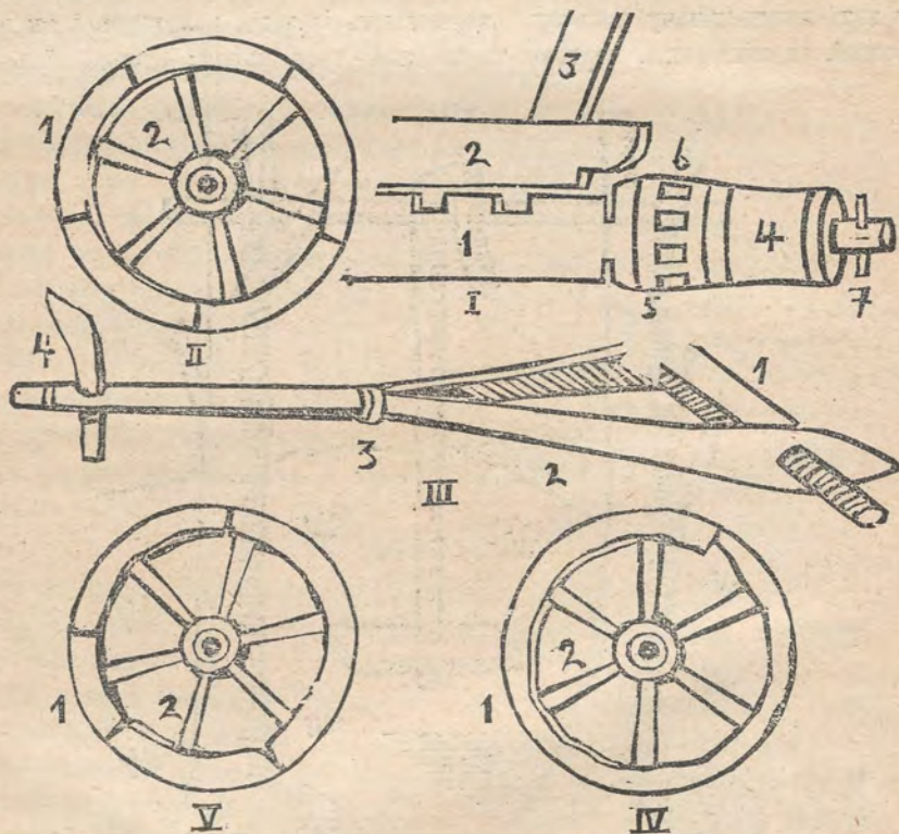
Рис. X. I. — 1 = снасть; 2 = насад; 3 = кляуак; 4 = колодка; 5 = обручка; 6 = гари; 7 = сторожка;
