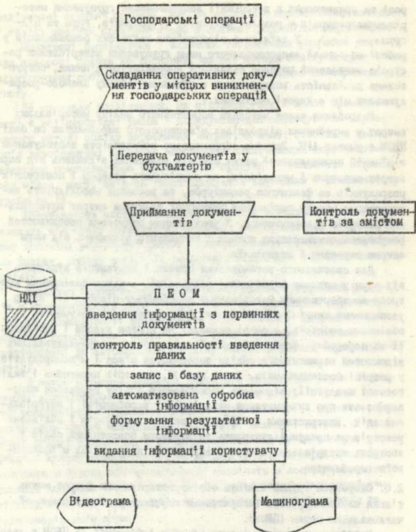
Мал. 1. Технологічний процес обробки об'єктові інформації в умовах АРМ
