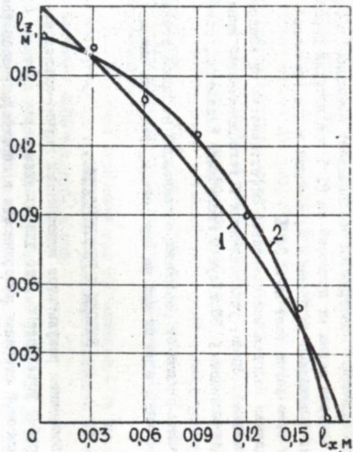
Рис. 4. Кривые осаждения зерен гречихи в сплавной камере: 1 - теоретическая; 2 - экспериментальная.
