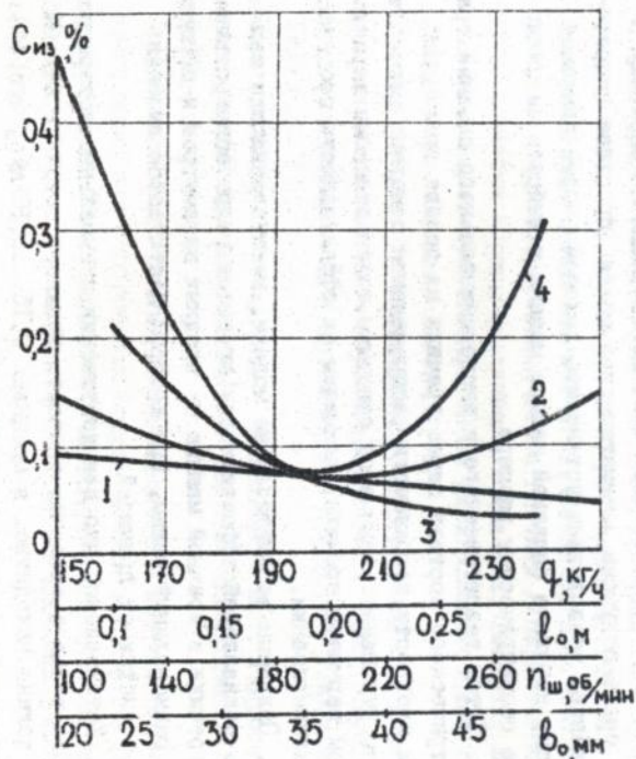
Рис. 3. Зависимость показателя C_{из} от параметров q (1); n_{ш} (2); l_0 (3); v_0 (4)
