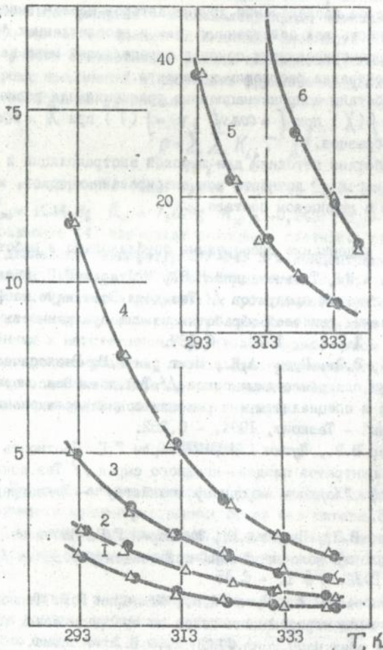
Рис. 1. Температурная зависимость вязкости яблочного и виноградного соков
