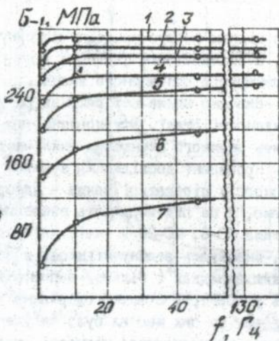
Рис.3. Вплив ПАР у обезвоженому мастилi MC-20 на опiр вто- мi сталi УВА в залежностi вiд її твердiстi
