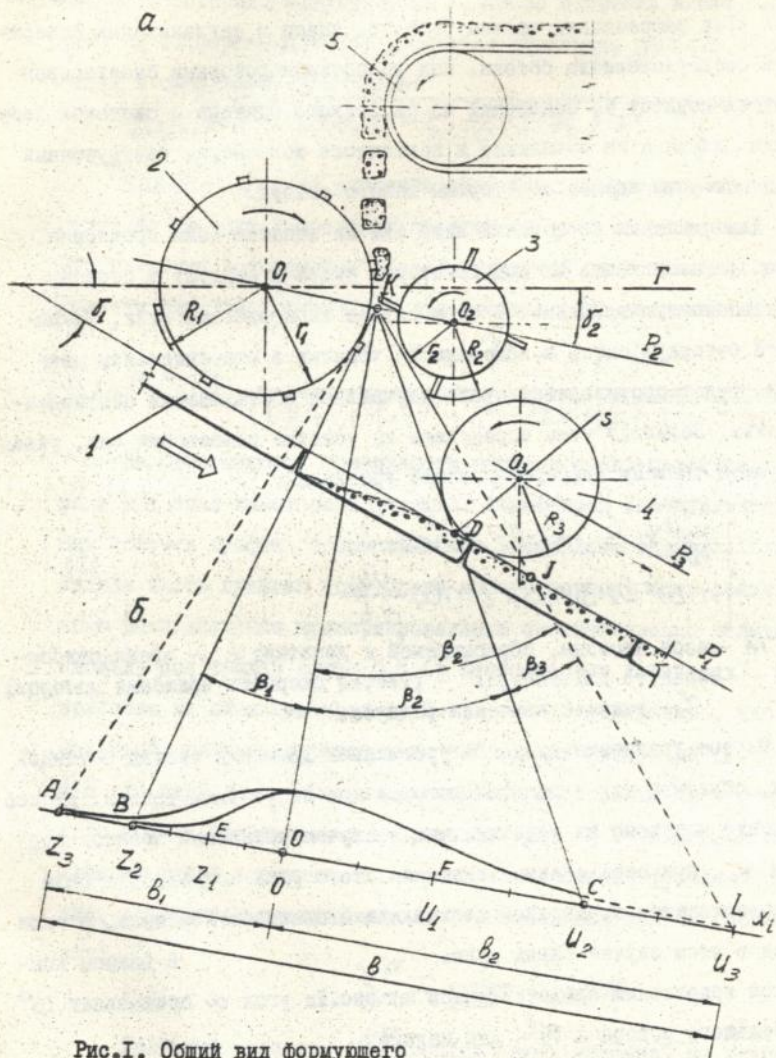
Рис. I. Общий вид формующего устройства
