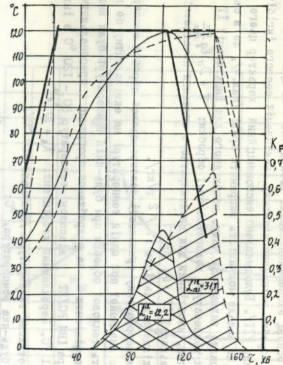
Мал. 5 Мікробіологічні і термодинамічні характеристики діючого і нового режимів стерилізації
