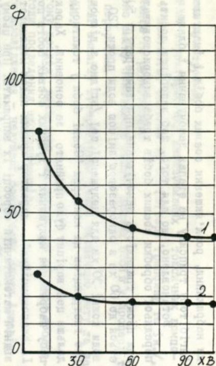
Мал.3 Характеристика розм'якшення сої при 60°C 1-Нелущена соя; 2-лущена соя
