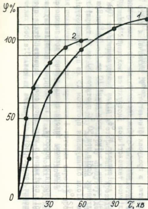
Мал.1 Характеристика набрякання сої при замочуванні при 60°C 1-нелущена соя; 2-лущена соя
