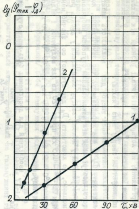
Мал.2 Криві інерції набрякання сої при замочуванні при 60°C 1-нелущена соя; 2-лущена соя
