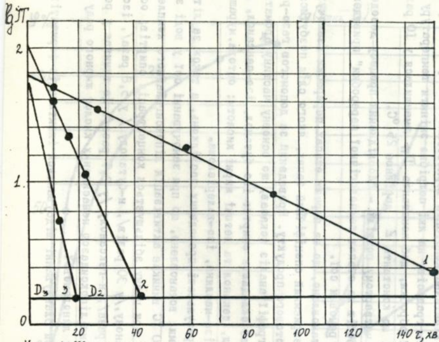
Мал. 4 Кінетика процесу інактивації соєвого інгібітору трипсину при вологотепловій обробці 1 - при 80°C; 2 - при 100°C; 3 - при 120°C
