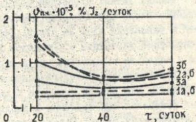
Рис.3. Динамика скорости изменения перекисного числа масел, хранившихся без доступа света при t = (4 \pm 1)^\circ\text{C} в закрытых (а) и открытых (б) емкостях
