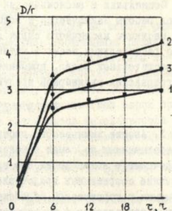
Рис.7. Динамика бензидинового числа жиров в процессе жарки
