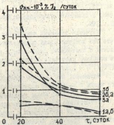
Рис.2. Динамика скорости изменения перекисного числа масел, хранившихся без доступа света при t = (20 \pm 1)^\circ\text{C} в закрытых (а) и открытых (б) емкостях
