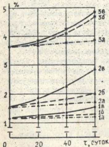
Рис.1. Динамика скорости изменения перекисного числа масел, хранившихся во свете при t = (20 \pm 1)^\circ\text{C} в закрытых (а) и открытых (б) емкостях
