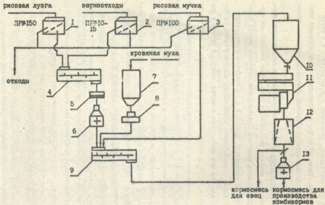
Рис. 4. Схема технологического процесса производства кормосмесей на рисоуаводе:
