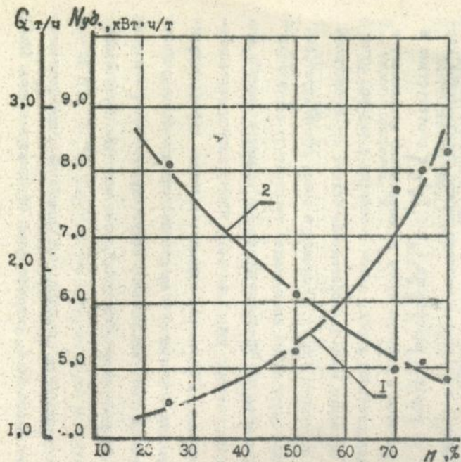
Рис.2. Зависимость производительности (I) молотковой дробилки А1-ДМР-6 и удельных энергозатрат на измельчение (2) от содержания зерноотходов в смеси с лузгой (n %).
