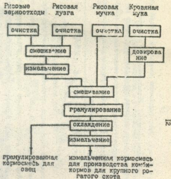
Рис.3. Постатная схема технологического процесса производства кормовых смесей из отходов переработки риса
