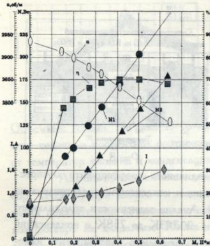
Рис.5. Характеристики электродвигателя ДАО 130-100.
