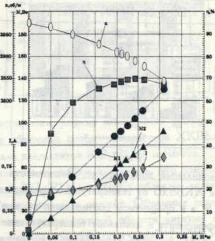
Рис.6. Характеристики электродвигателя ДАО 130-60.
