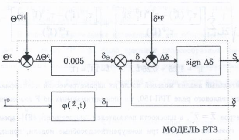
Рис. 1. Структурная схема модели РТЗ
