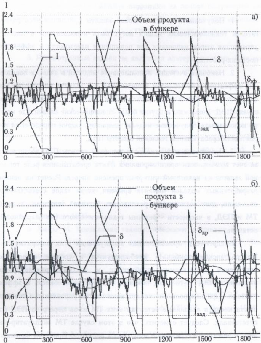
Рис. 4. Фрагмент результатов моделирования "обычной" САР и САР с коррекцией заданного значения тока
