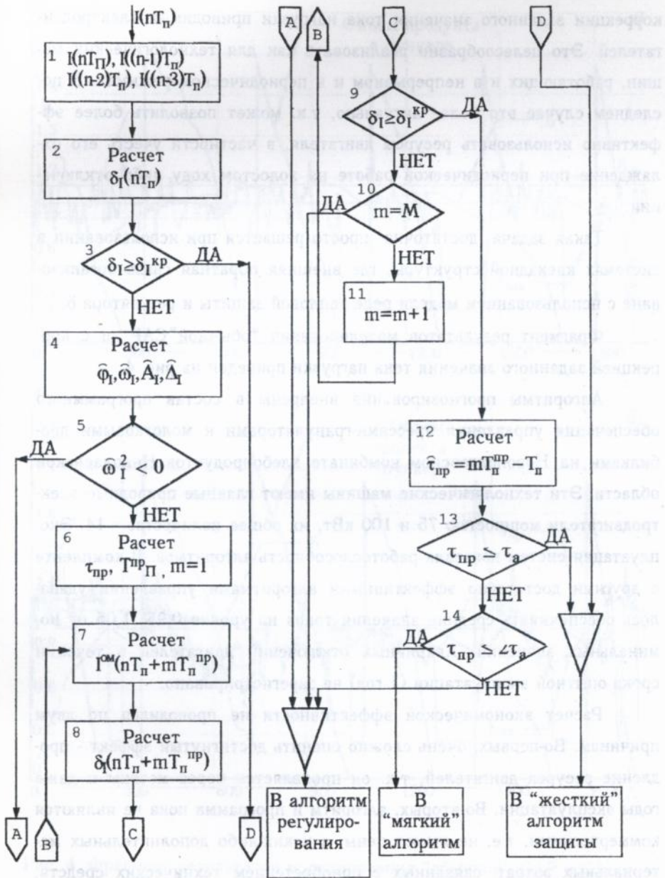
Рис. 3. Блок-схема алгоритма прогнозирования срабатывания РТЗ
