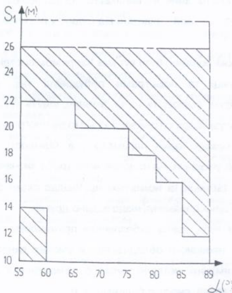
Рисунок 6 - Номограма до завдання 2 (постріл через будинок): закреслена зона - мета досягнута ( в таблиці - "1"); незакреслена зона - мета не досягнута ( в таблиці - "0").
