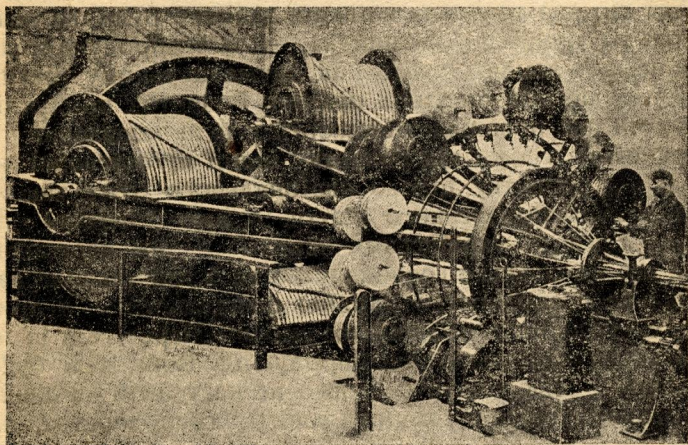
Машина, що продукує грубий дріт.
