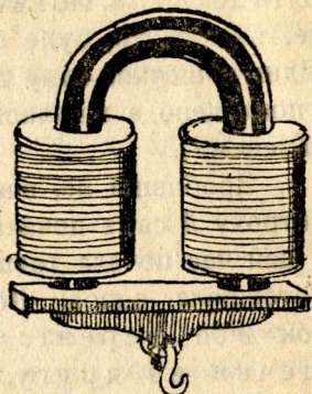
Електромагніт.
