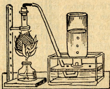
Рис. 8. Добування кислороду.
