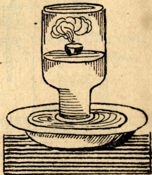
Рис. 9. Добування азоту.
