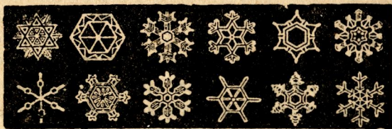
Рис. 4. Сніжинки.
