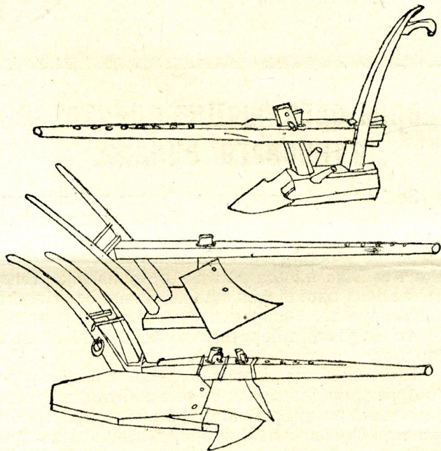
Обр. 1. рало. 2. рухадло. 3. зліпшене рало (плуг).
