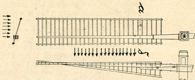
Рис. 3. Крило чотирокрилового вітряка; на ліво нарисоване крило так, як його бачимо з переду, на право так, як бачимо його з боку, а на долі нарисоване положення ребра в місці означенім буквами а—б. Стрілки означають напрям вітру.
