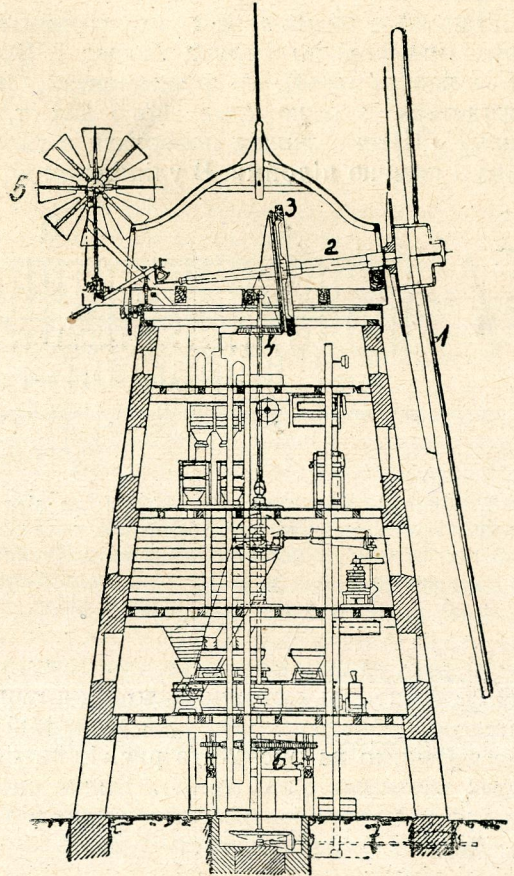
Рис. 2. Переріз більшого вітрового млина без галерії: 1 — крила проміром 23 м.; долішні кінці крил 3 м. від землі. — 2 — вісь крил, як видно з цього рисунку, а також з рисунку 1, не лежить поземі, але є наклонена під кутом 6—15° до поземі. — 3 — велике зубчате коло проміром 343 см. на осі крил; до нього прищурбований деревляний перстень (зараз біля цифри 3), що його може стискати прикріплений до бальків обруч; це ж і гальма, щоби можна було вітряк задержати коли треба. Від обруча йде підойма поза „шапку“ на двір а від неї тягло на довину; підойму і тягло видно з лівої сторони на рис. 1. — 4 — мале зубчате коло на доземому валі. — 5 — два помічні вітрячки по обох боках вала (на рисунку видно тільки один, бо другий, перед ним, „відрізаний“ з передною половиною будинку). Промір вітрячків 3 м. — велике зубчате коло на долі, що зачіпає за зуби зубчатих коліс на трьох веретенах млинських каменів. — Щоби млин на випадок ушкодження горішнього механізму, чи з браку вітру, не мусів стояти, можна його пнати паровою машиною чи иншим мотором з помічу вала „7“ та пари стійкових коліс.
