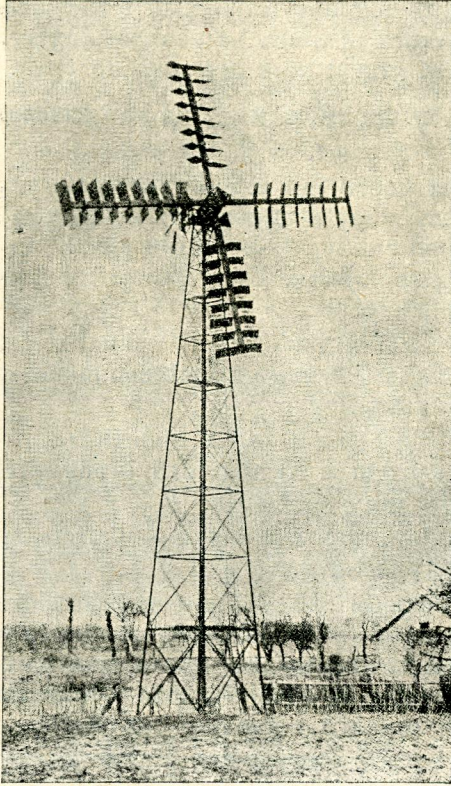
Рис. 6. Тут бачимо, як під напором надто сильного вітру поодинокі частини крил повернулись. Таке саме уладження має вітряк на рис. 1. Там можна „поотвирати“ усі кляпи ручно з помічно підойми або ланцюхів на зовні будинку. Роблять це тому, щоби вітряк (т. є. його крила) не був виставлений на тис- нення вітру, якщо він не має працювати.
