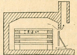
Сушарня в печі.
