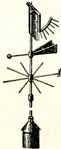
Рис. 7. Прилад до мірвання швидкості вітру.
