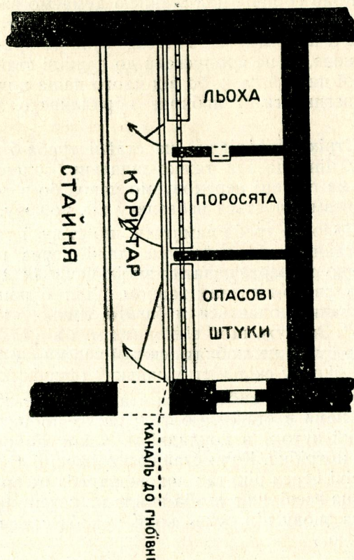
Плян стайні.
