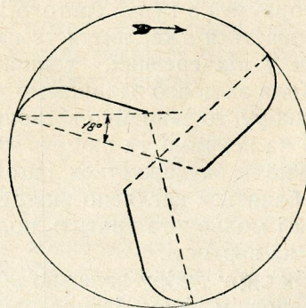
Рис. 11. Показує у погляді з гори, яку форму мають лопатки вітряка на рис. 10.
