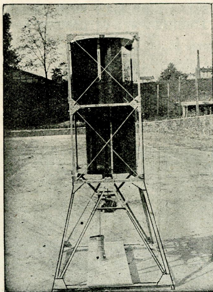
Рис. 12. Модель вальцевого вітряка з трьома лопатками і двома вальцями на низькій залізній вежі для цілей меліорації.
