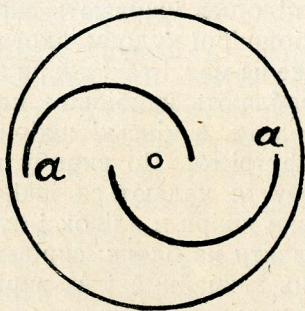
Рис. 9. Цей рисунок показує у погляді згори, як вигнуті є дві півкругові вальцеві лопатки вітряка Савоніюса.
