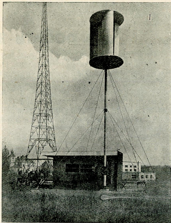
Рис. 10. Вальцевий вітряк з трьома лопатками, що досі ще стоїть на площі Східних Торгів у Львові біля львівської радіостанції.
