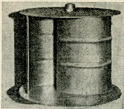
Рис. 8. Вальцевий (роторовий) вітряк систему інж. Савоніюса.
