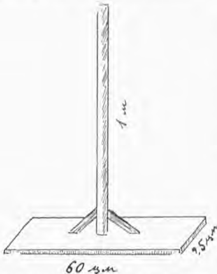
Стежкар, приряд до відмірювання стежок.
